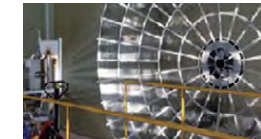
400kW급 KIER 태양로 (바이오메탄 분해 수소생산 실험)
